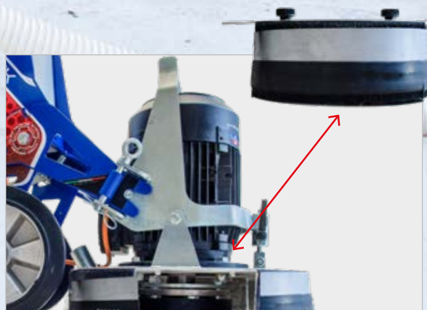
Sportello laterale removibile per legatura a filo
